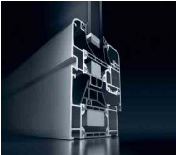
Schüco Fenster AWS 70 SL.HI Abgerundete Soft Line-Flügelkontur für eine weiche Linienführung Schüco window AWS 70 SL.HI Rounded Soft Line vent contour for soft lines
